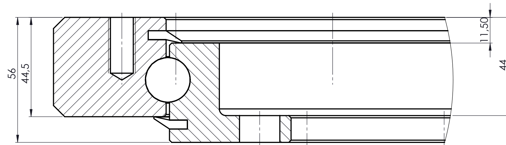
DETAIL B MAßSTAB 1 : 1
