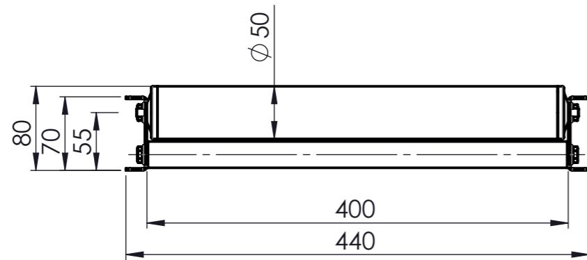
Ansicht A 1:5
