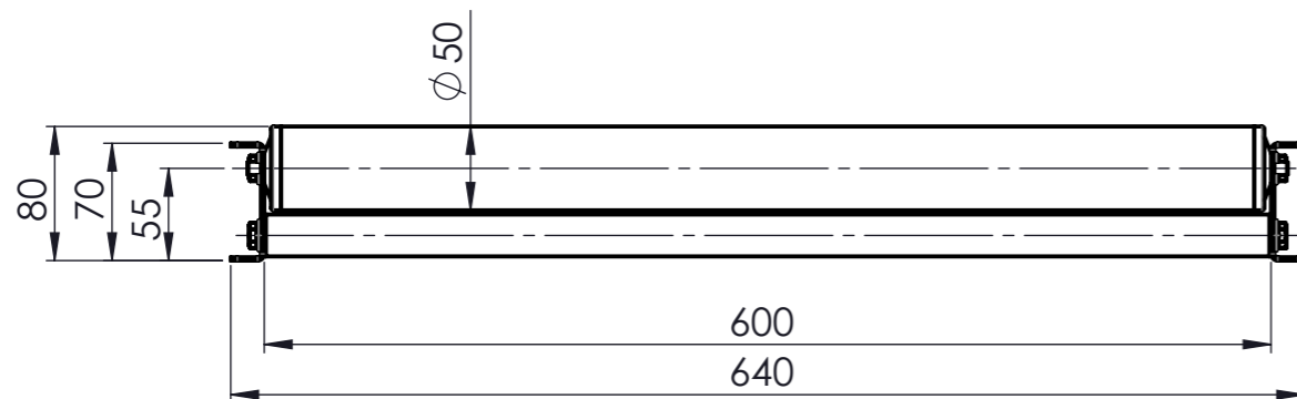
Ansicht A 1:5
