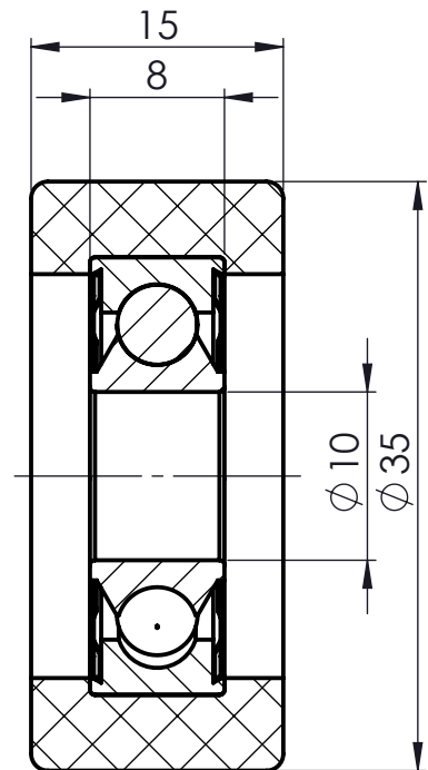
SCHNITT A-A
