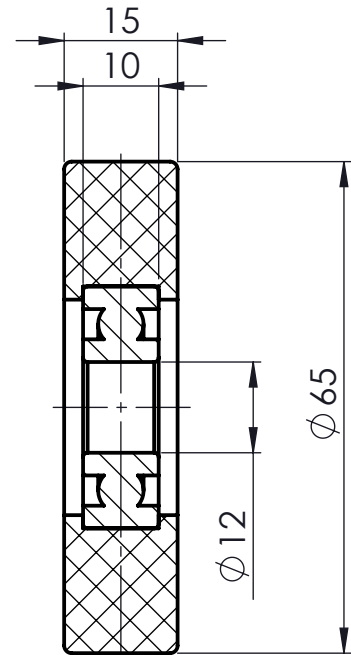
SCHNITT A-A
