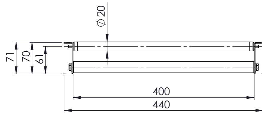
Ansicht A 1:5
