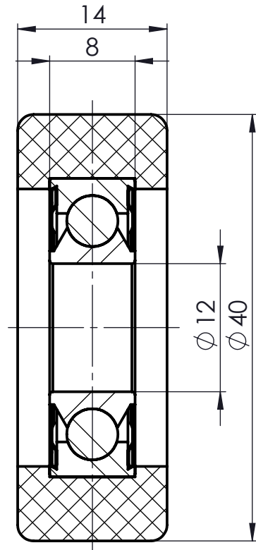
SCHNITT A-A
