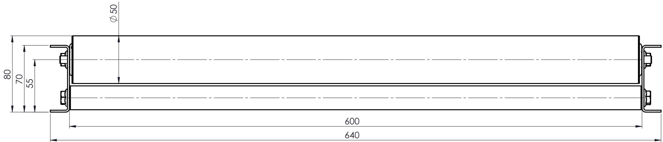
Ansicht A
