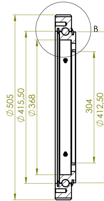
SCHNITT A-A
