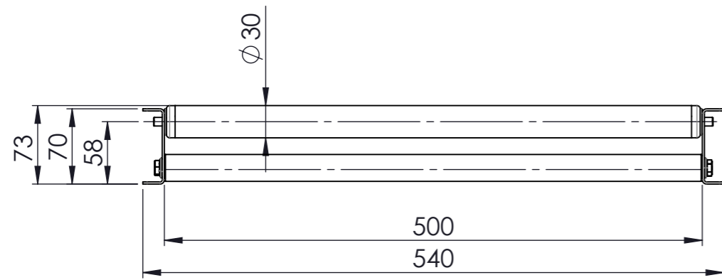
Ansicht A 1:5
