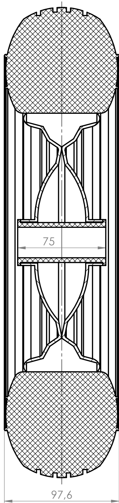
SCHNITT A-A
