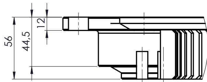
DETAIL B MAßSTAB 1 : 2
