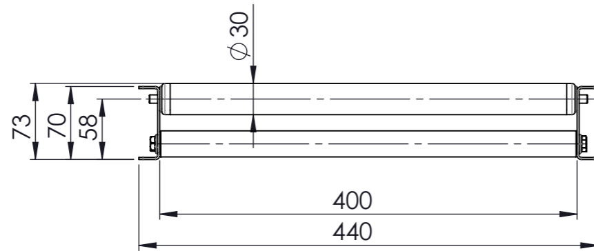
Ansicht A 1:5
