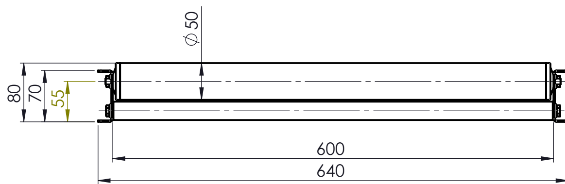
Ansicht A 1:5
