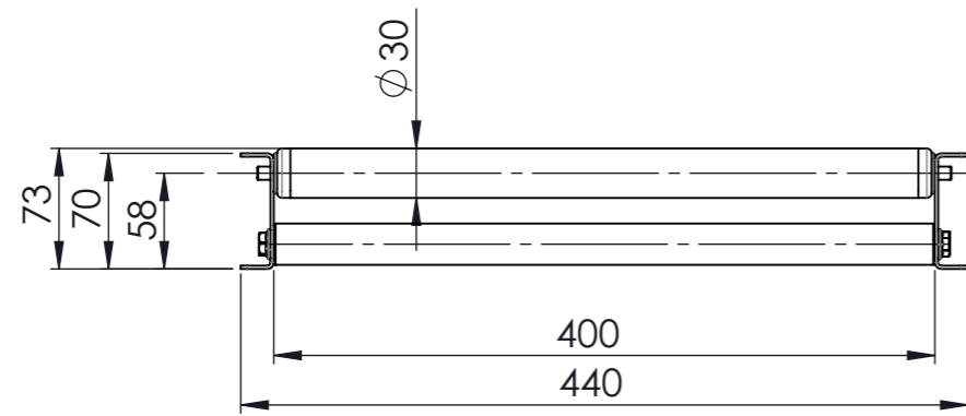
Ansicht A 1:5
