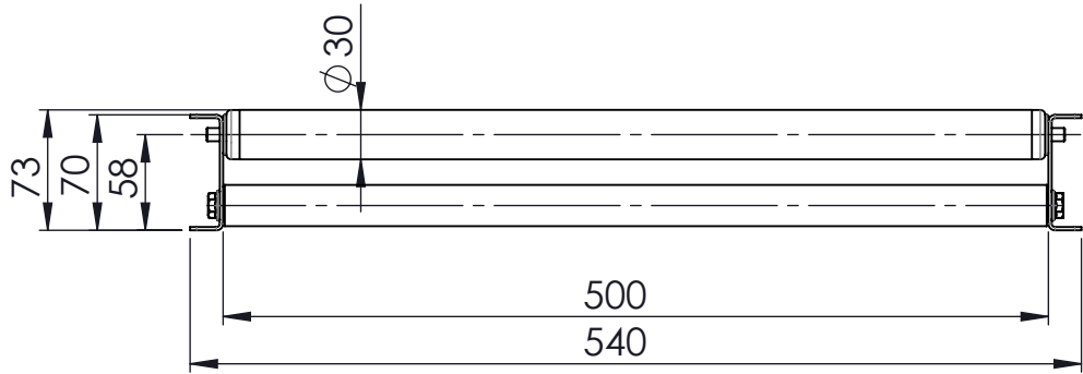
Ansicht A 1:5
