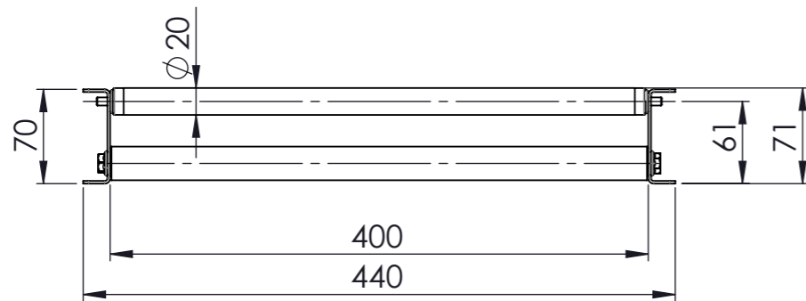
Ansicht A 1:5
