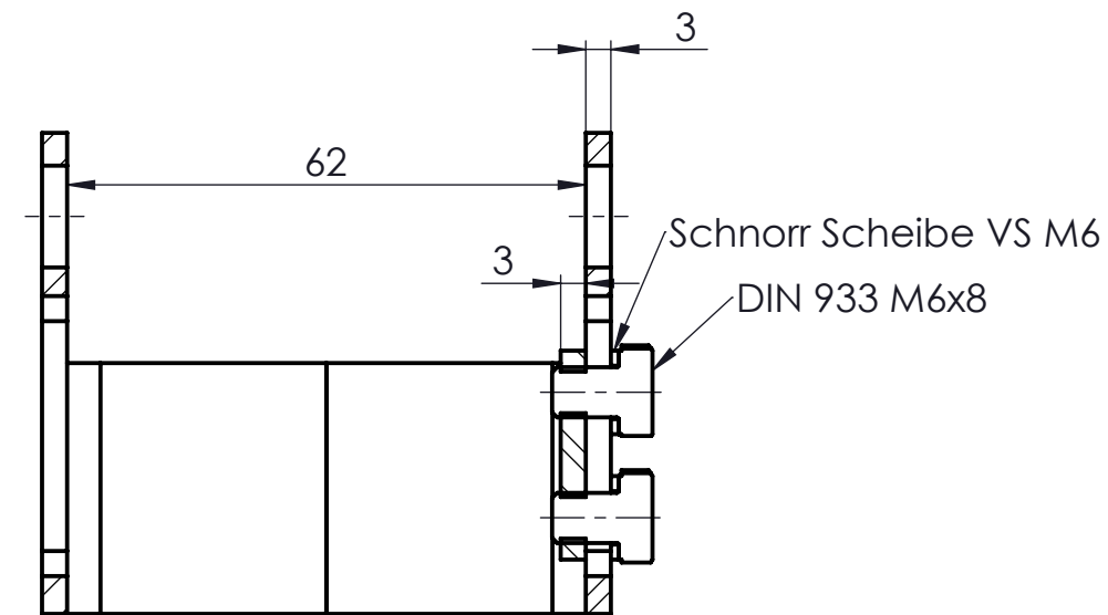
SCHNITT A-A
