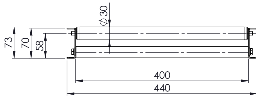
Ansicht A 1:5
