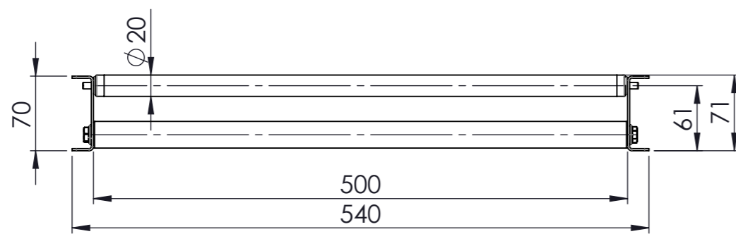
Ansicht A 1:5
