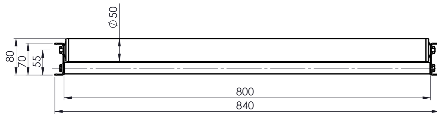
Ansicht A 1:5
