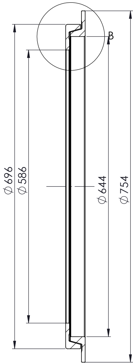
SCHNITT A-A
