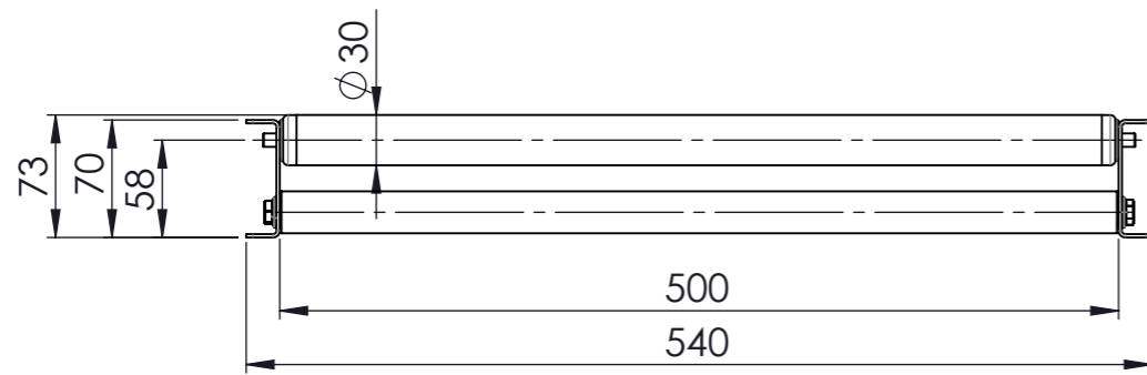
Ansicht A 1:5
