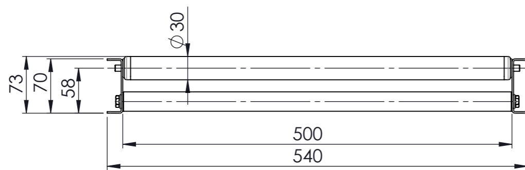
Ansicht A 1:5
