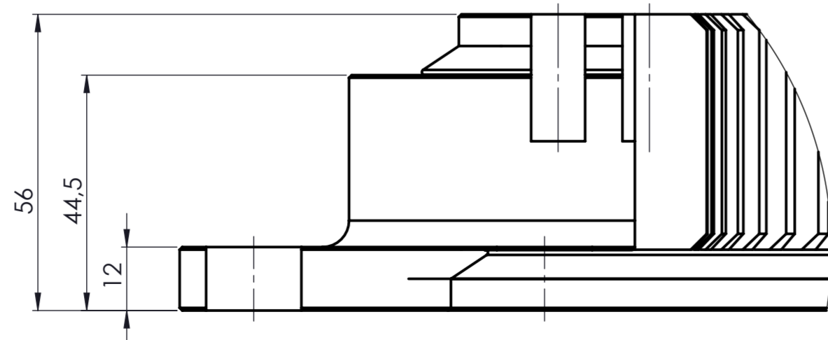
DETAIL B MAßSTAB 1 : 1
