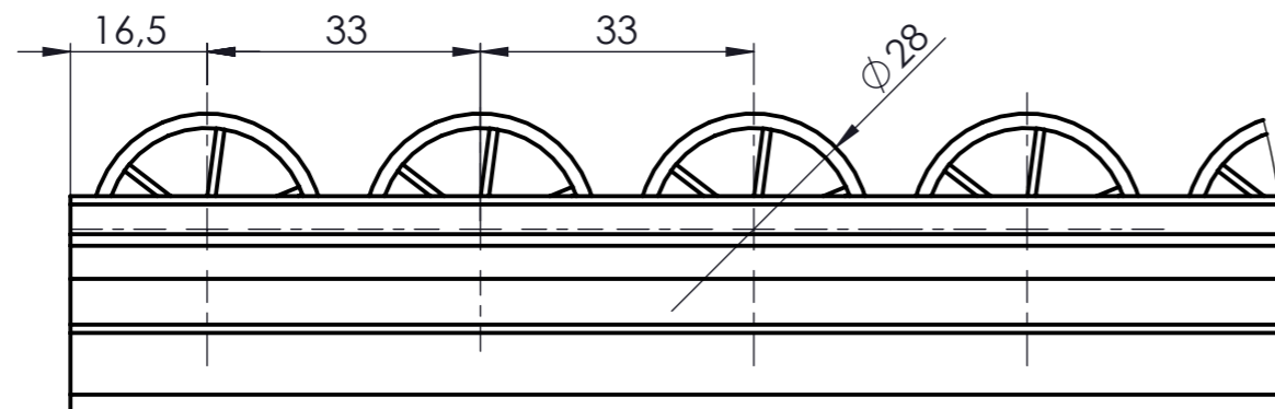
DETAIL B MAßSTAB 1 : 1
