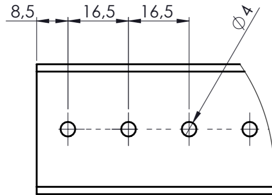
DETAIL A MAßSTAB 1 : 1
