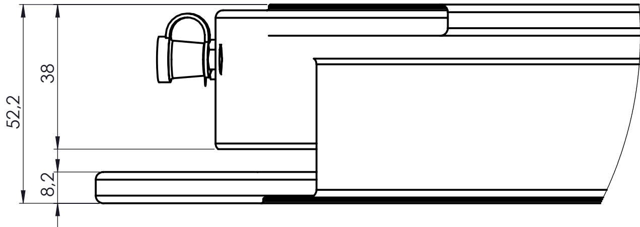
DETAIL B MAßSTAB 1 : 1
