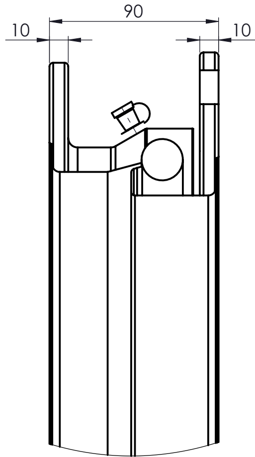
DETAIL B MAßSTAB 1 : 2
