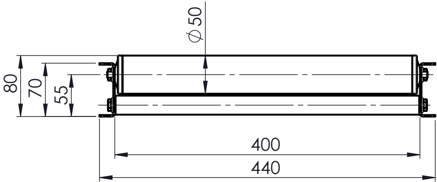
Ansicht A 1:5
