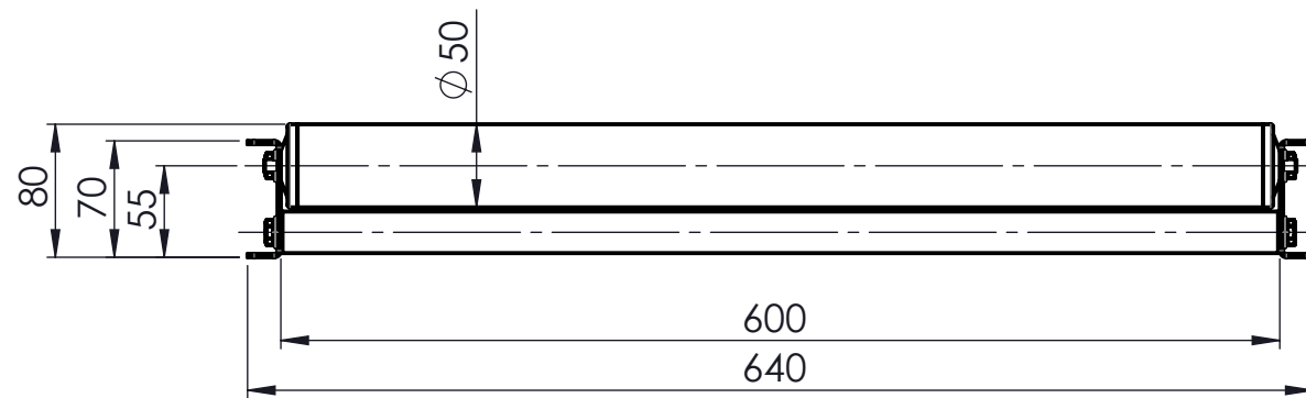
Ansicht A 1:5
