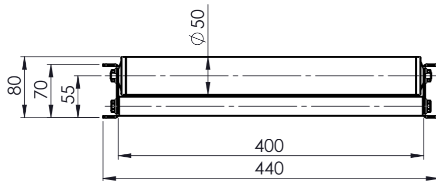
Ansicht A 1:5
