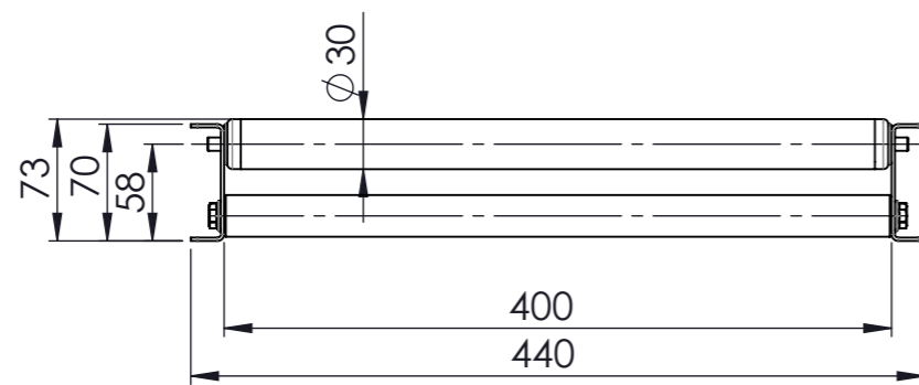
Ansicht A 1:5
