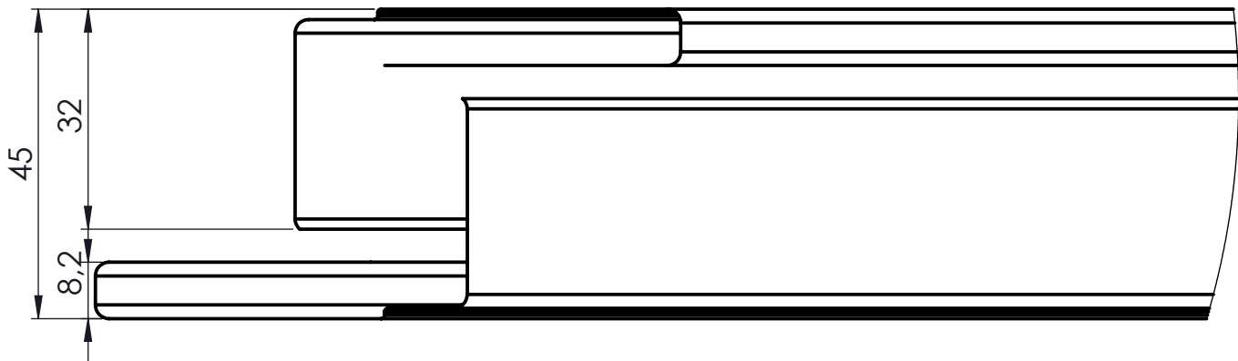
DETAIL B MAßSTAB 1 : 1
