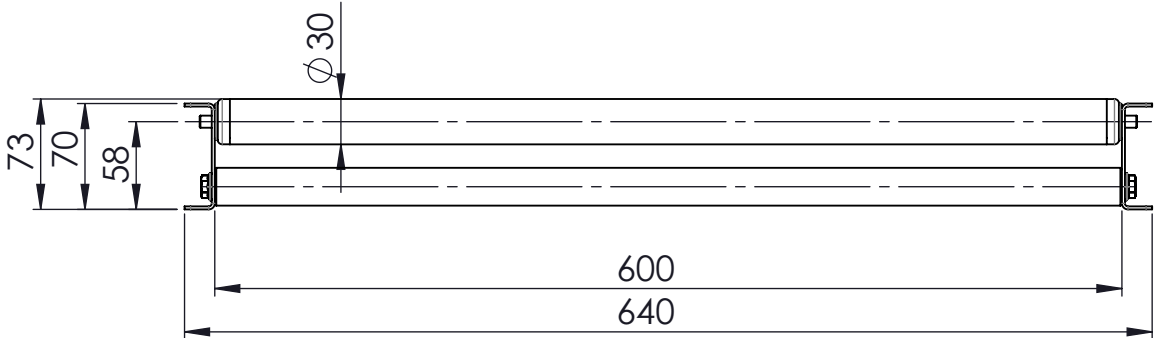
Ansicht A 1:5
